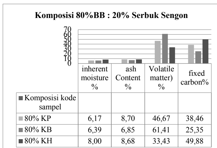
Gambar 2. Grafik Analisis Proksimat Briket Pada Komposisi 80% : 20%
