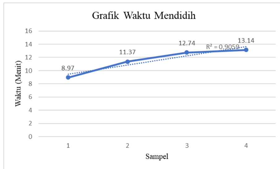
Gambar 1. 2 Grafik pengaruh penambahan kulit durian terhadap waktu mendidihkan air
